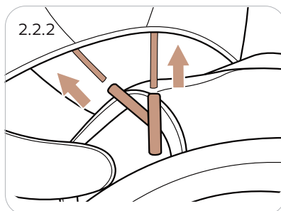
2.2.2 Trek de steun van de kap (14) aan beide zijden uit de zwarte buis.
